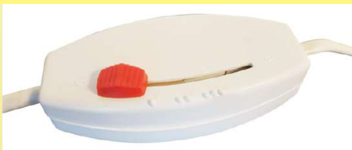
Interruptor calefactor de 3 posiciones y interruptor de apagado de 2 posiciones en manta térmica. Modelo intermedio entre sistemas rotativos y sistemas deslizantes (Circa 1970. Colección Gitem Ultimheat)
