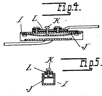
1912 Termostato bimetalico Hoffmann para manta térmica (Patente estadounidense 1096916). J es una hoja bimetalica remachada en ambos extremos. Se supone que el contacto eléctrico se abrirá entre la hoja J, deformándose cuando la temperatura sube, y el tornillo de ajuste K.
