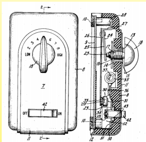
Sistema para regular la potencia de mantas calefactoras bimetálicas y resistencia adicional en la carcasa (1942, patente de Cook)
