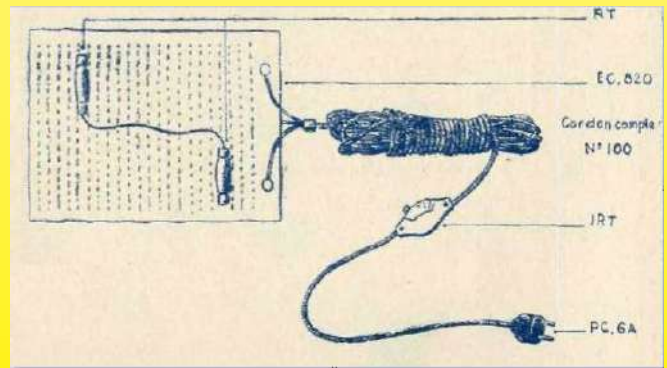
1947 Calor Thermoplasma, vista de la parte calefactora con sus termostatos protegidos (RT) y su interruptor de 3 posiciones (IRT). (Catálogo Ultimheat)
